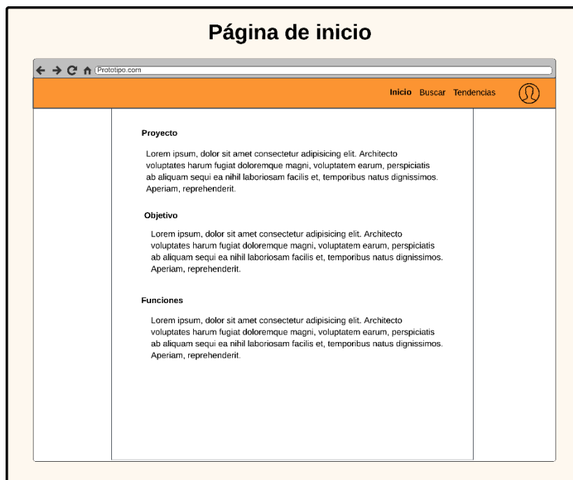
Ilustración 2: Página inicial
