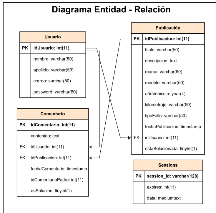
Figura 3: Diagrama Entidad-Relación
